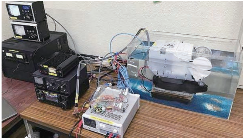
海中ワイヤレス給電の実験（同）
